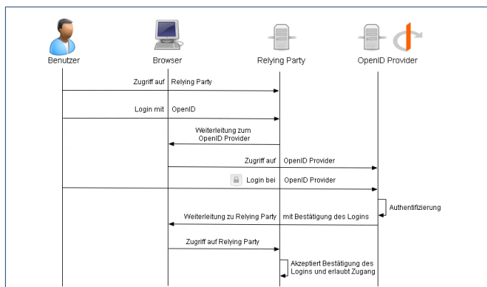
Der Ablauf des Authentifizierungsvorgangs mit OpenID.
